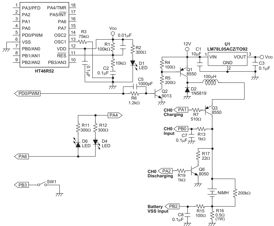
充电器应用电路图
